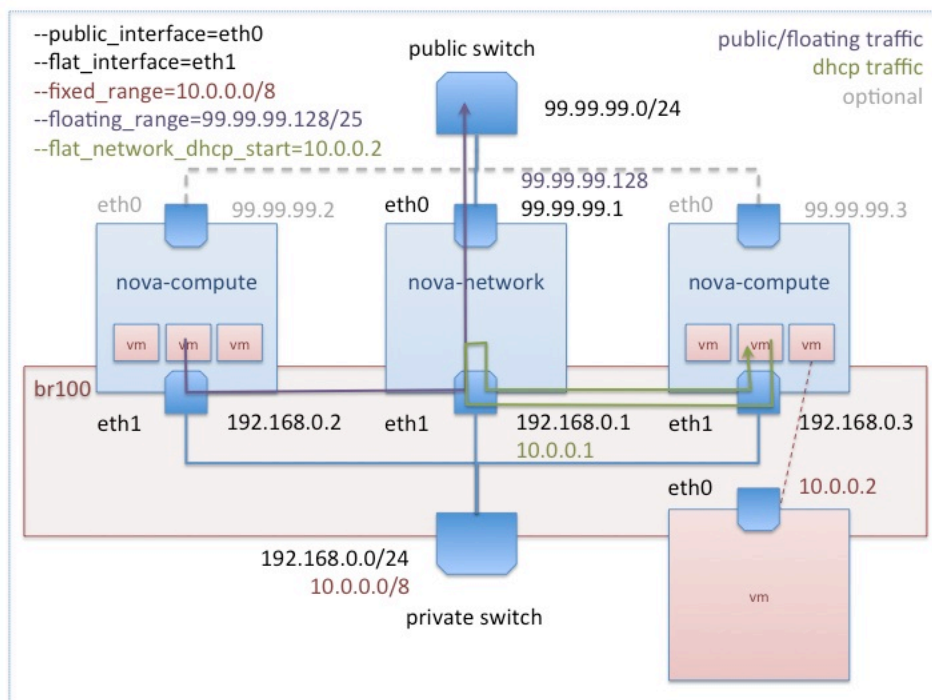
Figura 5.4. Flat DHCP network con libvirt, múltiples interfaces y múltiples servidores
